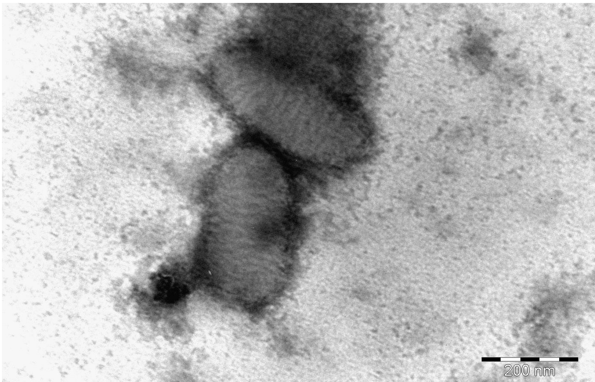
TEM Bovines Parapoxvirus, charakteristische wollknäulartige Innenstruktur
